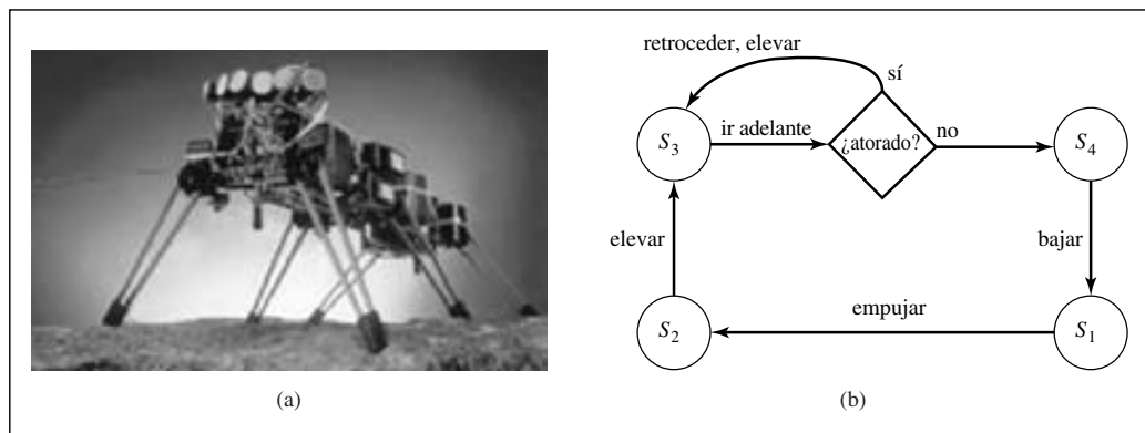
Figura 25.22 (a) un robot hexápodo (b) Un autómata finito aumentado (AFSM o augmented finite state machine ) para el control de una única pierna. Este AFSM reacciona a la retroalimentación de los sensores: si una pierna se atasca durante la fase de movimiento hacia delante, se elevará incrementalmente.
