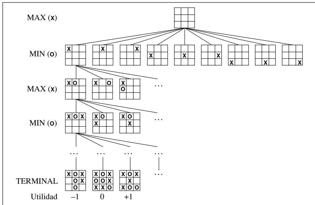
Figura 6.1 Un árbol (parcial) de búsqueda para el juego de tic-tac-toe. El nodo de arriba es el estado inicial, y MAX mueve primero, colocando un X en un cuadrado vacío. Mostramos la parte del árbol de búsqueda, con movimientos alternados por MIN (O) y MAX, hasta que finalmente alcancemos estados terminales, en los cuales podemos asignar utilidades según las reglas del juego.
