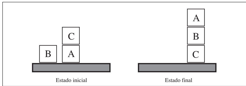
Figura 11.16 El problema de planificación «anomalía de Sussman» en un mundo de bloques.
