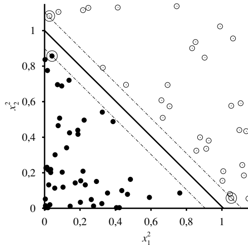
Figura 20.28 Un plano, proyectado en la primera de las dos dimensiones, del separador óptimo mostrado en la Figura 20.27(b). El separador se muestra como una línea realzada, con los puntos más cercanos (los vectores soporte ) marcados con círculos. El margen es la separación entre los ejemplos positivos y los ejemplos negativos.
