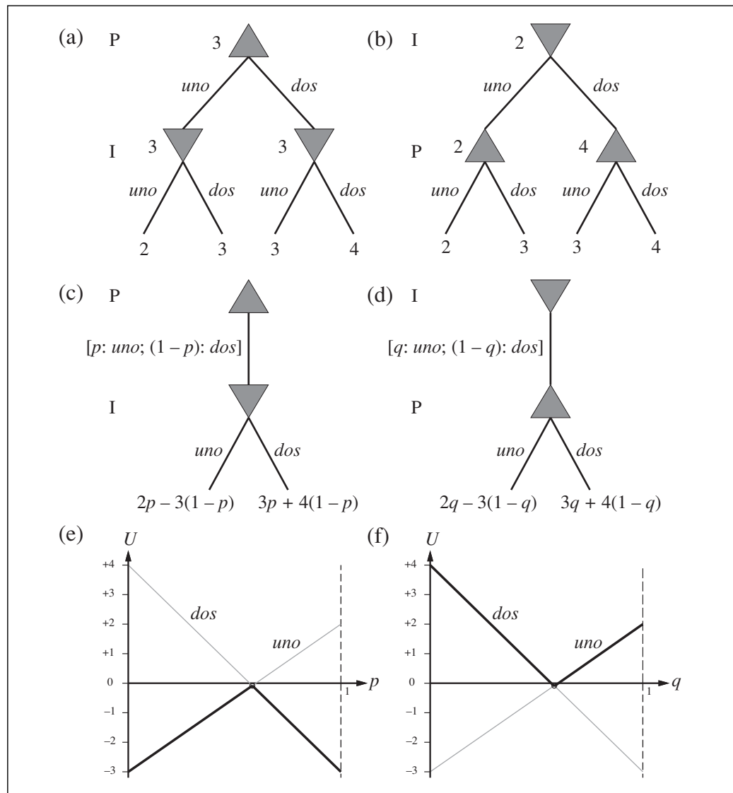
Figura 17.11 (a) y (b): árboles minimax para el juego «pares o noes» si los jugadores juegan por turno estrategias puras. (c) y (d): árboles parametrizados del juego en los que el primer jugador juega una estrategia mixta. Los balances finales dependen de la probabilidad del parámetro ( p o q ) de la estrategia mixta. (e) y (f): para cada valor particular de probabilidad, el segundo deberá elegir la «mejor» de las dos acciones, de forma que el valor de la estrategia mixta del primer jugador viene dada por los tramos gruesos. El primer jugador elegirá como valor del parámetro la probabilidad de la estrategia mixta en el punto de intersección.
