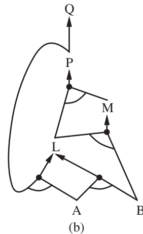
Figura 7.15 (a) Una base de conocimiento sencilla con cláusulas de Horn. (b) Su correspondiente grafo Y-O.
