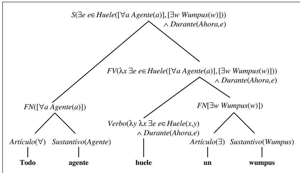
Figura 22.19 Árbol de análisis gramatical para la oración «Todo agente huele un wumpus», mostrando tanto la interpretaciones semánticas como la estructura sintáctica.
