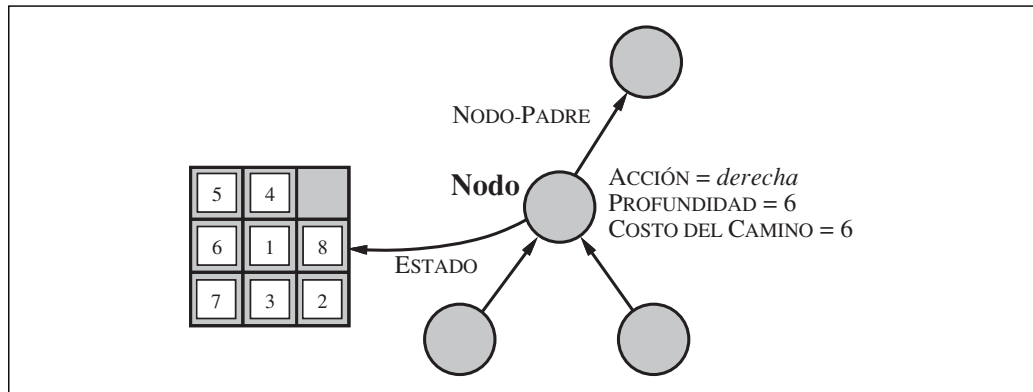
Figura 3.8 Los nodos son estructuras de datos a partir de los cuales se construye el árbol de búsqueda. Cada uno tiene un padre, un estado y varios campos. Las flechas señalan del hijo al padre.
