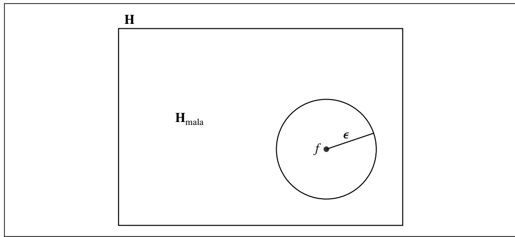
Figura 18.12 Diagrama esquemático del espacio de hipótesis, mostrando la zona que cubre la \epsilon -bola alrededor de la función f .
