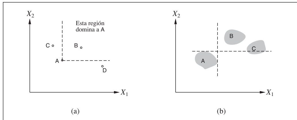
Figura 16.3 Predominio estricto. (a) Determinista: opción A está estrictamente dominada por la opción B pero no por C ni D. (b) Incertidumbre: A está dominada estrictamente por B pero no por C.
