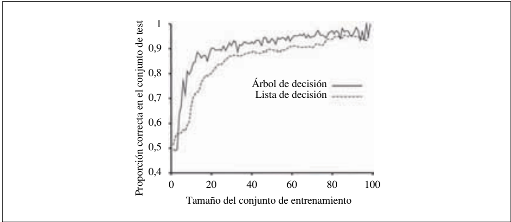
Figura 18.15 Curva de aprendizaje para el algoritmo APRENDIZAJE-LISTA-DECISIÓN sobre los datos del restaurante. La curva del algoritmo APRENDIZAJE-ÁRBOL-DECISIÓN se muestra para comparar.
