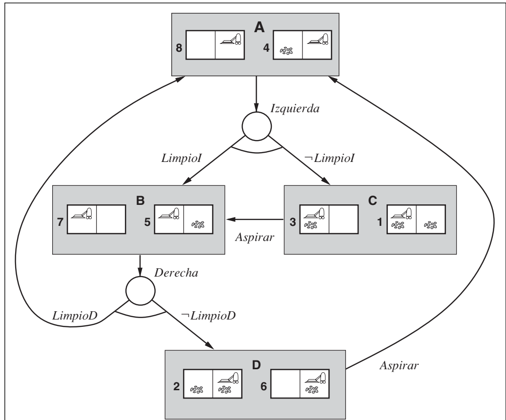
Figura 12.12 Parte del grafo AND-OR para el mundo aspiradora «doble Murphy recíproco», en el cual la suciedad puede a veces ser abandonada tras el agente cuando éste se mueve hacia una posición limpia. El agente no es sensible a suciedad en otras posiciones.
