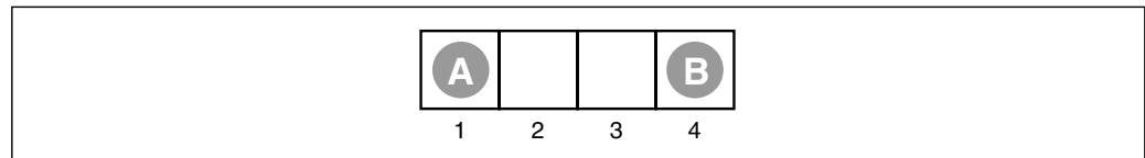
Figura 6.14 La posición de partida de un juego sencillo. El jugador A mueve primero. Los dos jugadores mueven por turno, y cada jugador debe mover su señal a un espacio vacío adyacente en una u otra dirección. Si el adversario ocupa un espacio adyacente, entonces un jugador puede saltar sobre el adversario al siguiente espacio vacío si existe. (Por ejemplo, si A está sobre 3 y B está sobre 2, entonces A puede mover hacia atrás a 1.) El juego se termina cuando un jugador alcanza el extremo opuesto del tablero. Si el jugador A alcanza el espacio 4 primero, el valor del juego a A es +1; si el jugador B alcanza el espacio 1 primero, entonces el valor del juego para A es -1.
