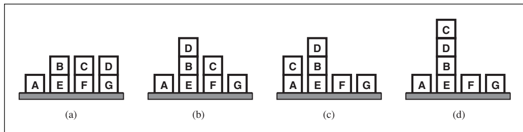
Figura 12.15 Secuencia de estados del agente de planificación continua que intenta alcanzar el estado objetivo Sobre(C, D) \wedge Sobre(D, B) , que se muestra en (d). El estado inicial es (a). En (b), otro agente ha interferido en el plan, colocando D sobre B . En (c), el agente ha ejecutado Mover(C, D) pero ha fallado, y ha colocado C sobre A . En la última fase reintenta Mover(C, D) , alcanzando el estado objetivo (d).
