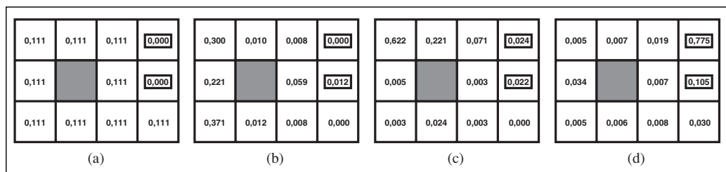
Figura 17.8 (a) Distribución de probabilidad inicial acerca de la localización del agente. (b) Después de moverse cinco veces a la Izquierda . (c) Después de moverse cinco veces Arriba . (d) Después de moverse cinco veces a la Derecha .
