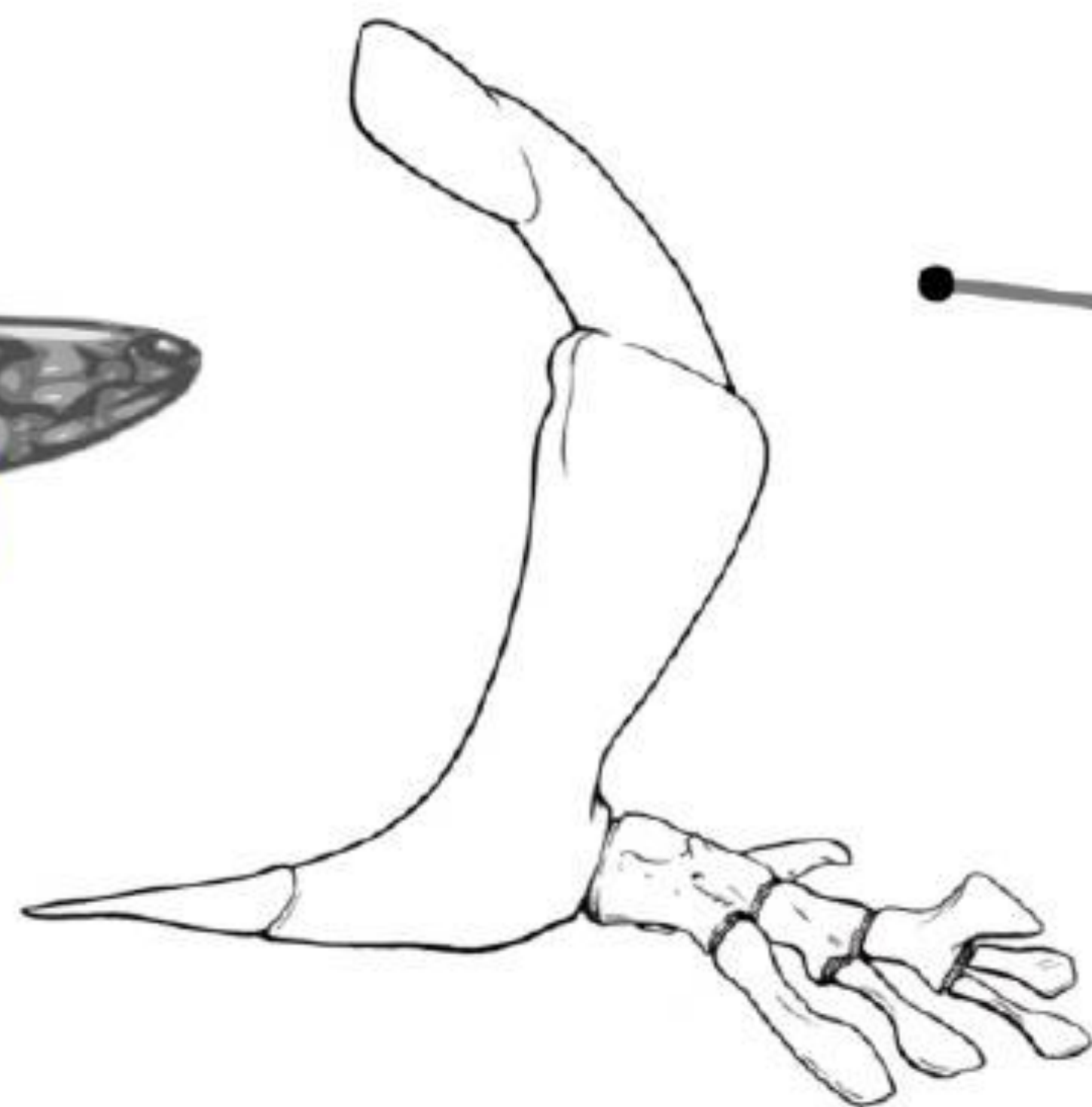
Eusthenopteron foordi †
