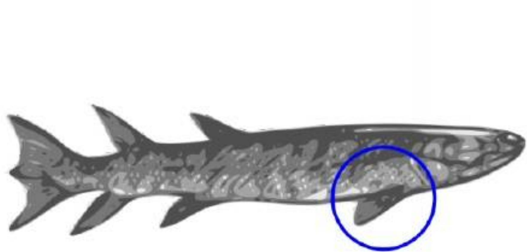
Eusthenopteron foordi †
